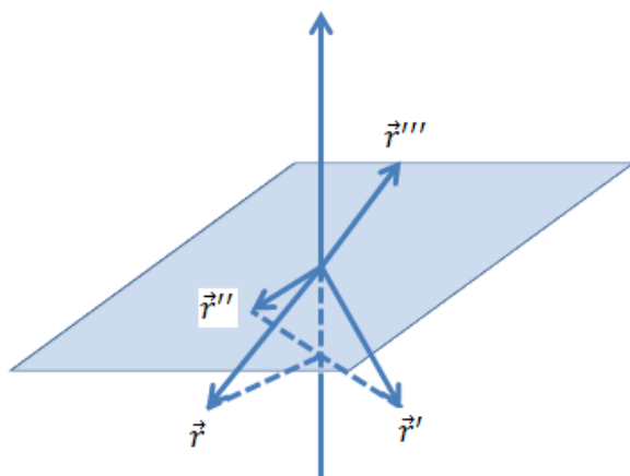
图 3.3 转动反演轴与转动反射面相互关系示意图
