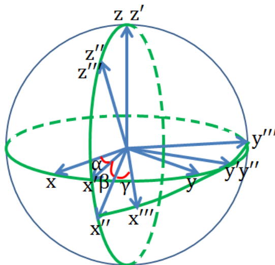
图 5.1 欧拉角
