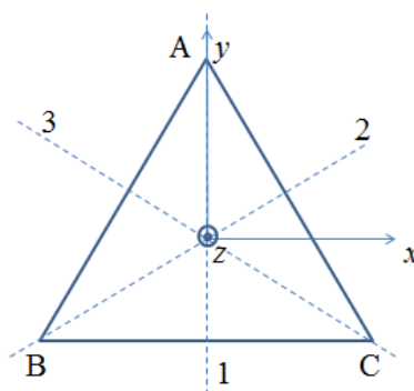
图 1.1 D_3 群示意图
