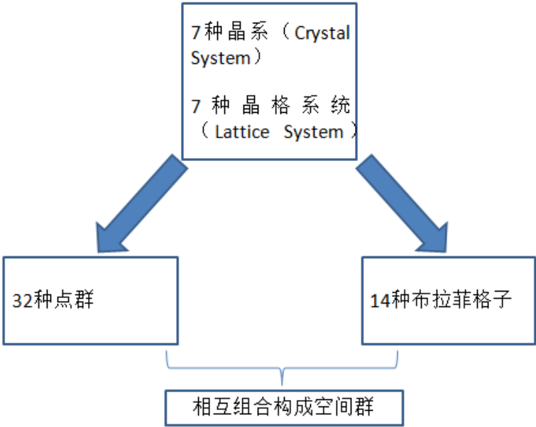
图 3.25 晶系、晶格系统、点群、布拉菲格子、空间群关系示意图
