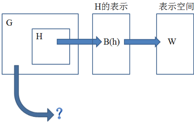
图 2.6 诱导表示示意图一
