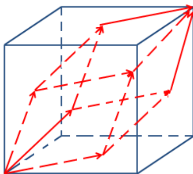
图 4.19 晶胞与元胞
