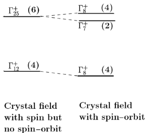
图 5.4 旋轨耦合引起的能级劈裂示意图
