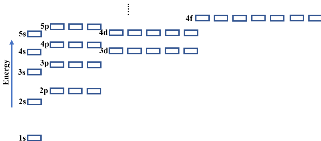
图 6.10 原子中的单电子轨道示意图
