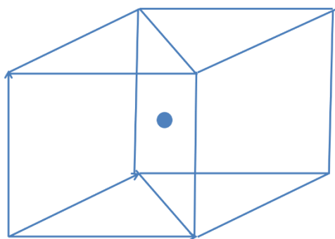
图 3.29 单斜格子中等价点示意图三
